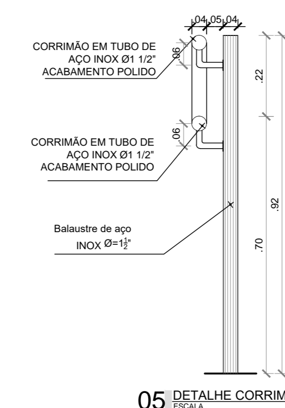
05 DETALHE CORRIMÃO
