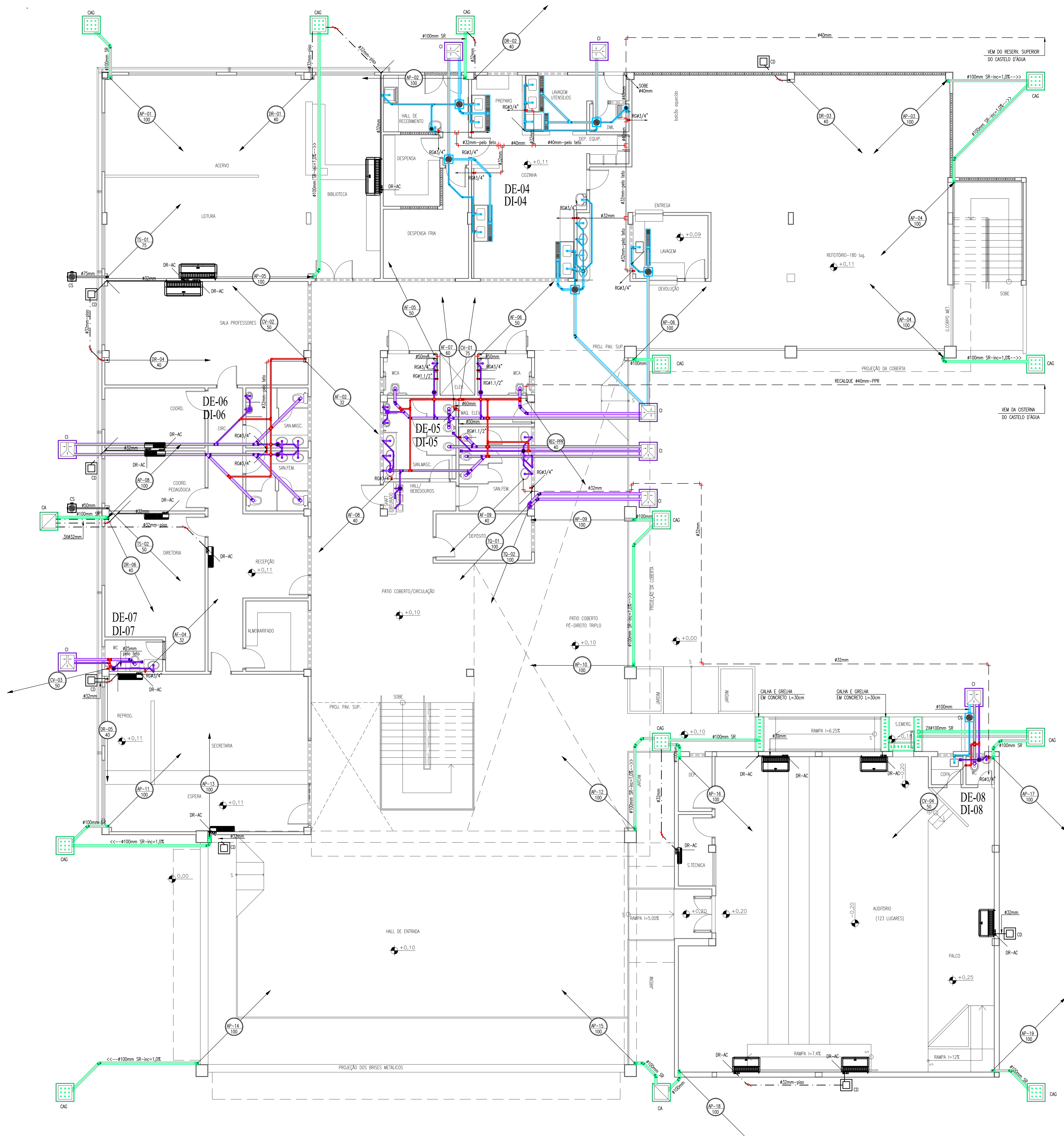
PLANTA PAV. TÉRREO ESCALA: 1/75
