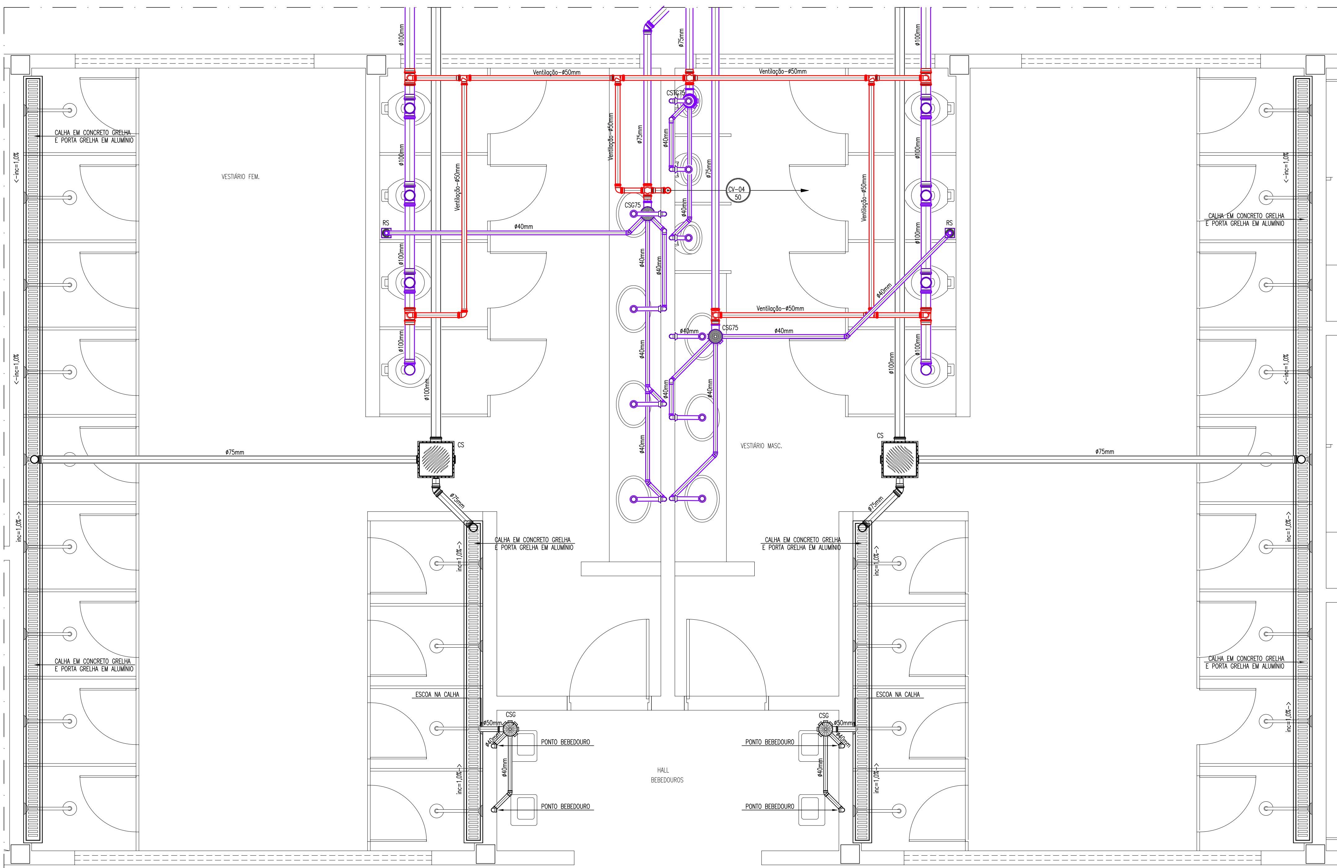
DETALHE DE ESGOTO 10 ESCALA: 1/25
