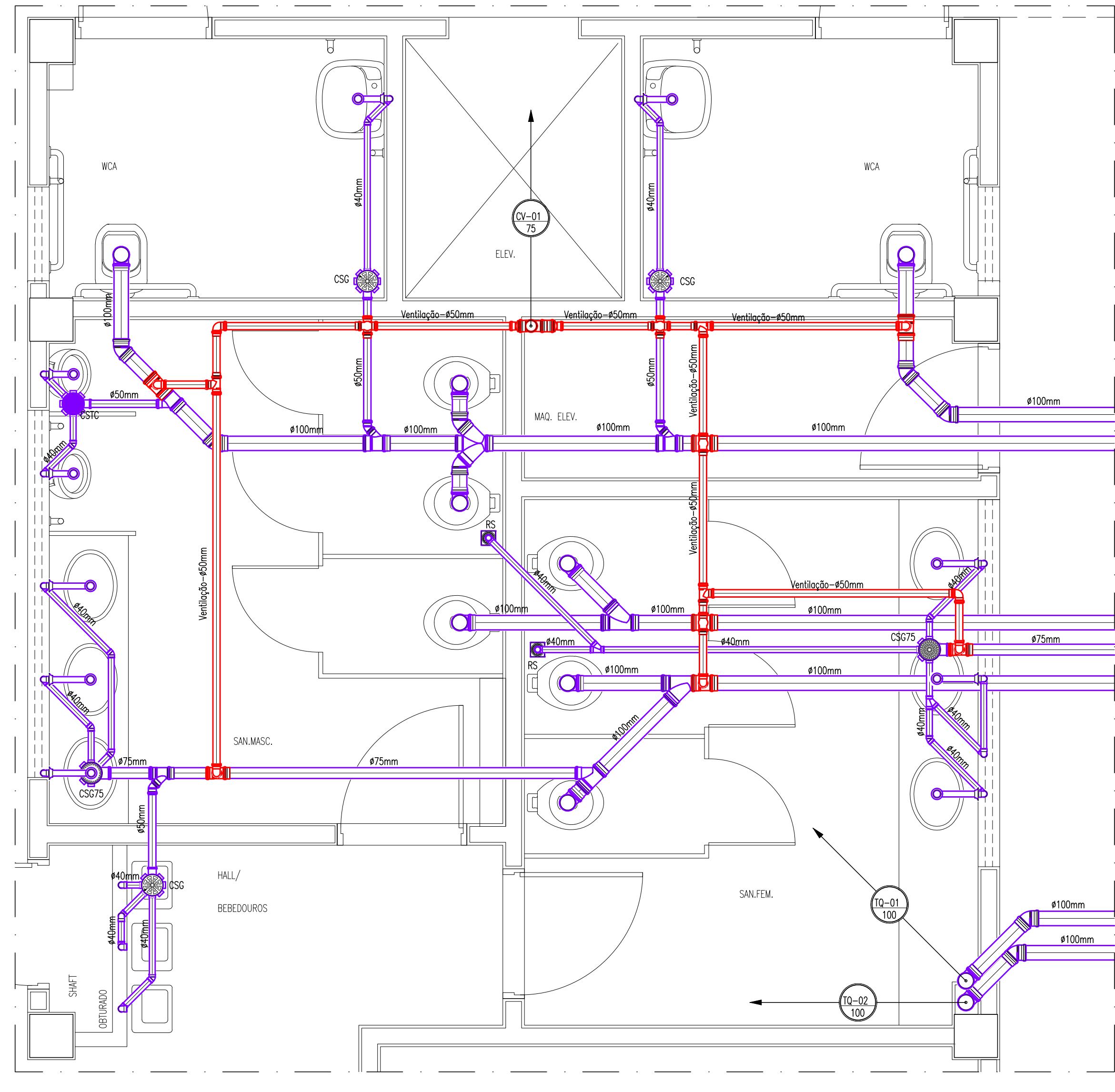
DETALHE DE ESGOTO 07 ESCALA: 1/25
