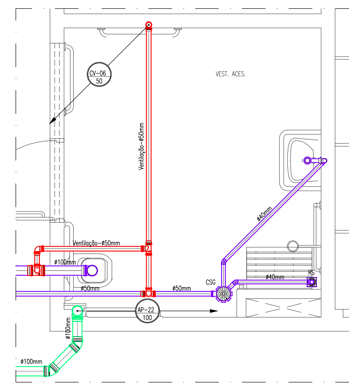
DETALHE DE ESGOTO 09 ESCALA: 1/25
