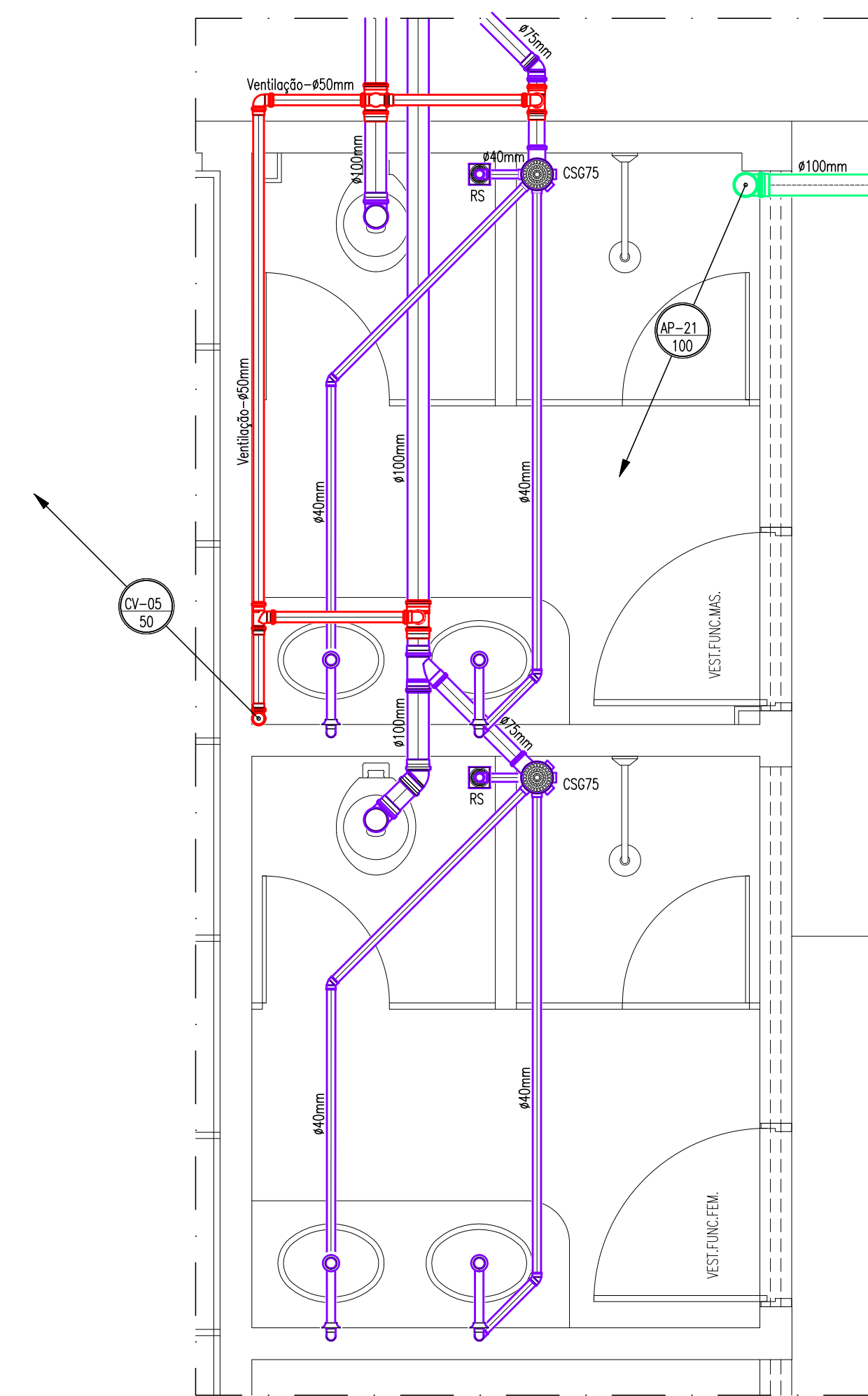
DETALHE DE ESGOTO 11 ESCALA: 1/25
