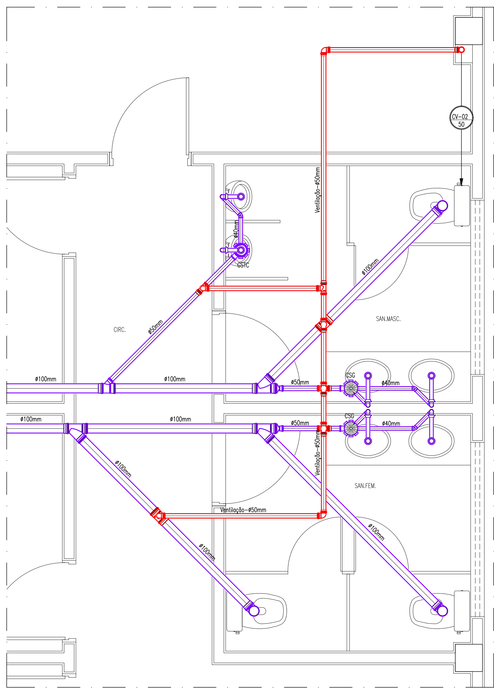
DETALHE DE ESGOTO 06 ESCALA: 1/25
