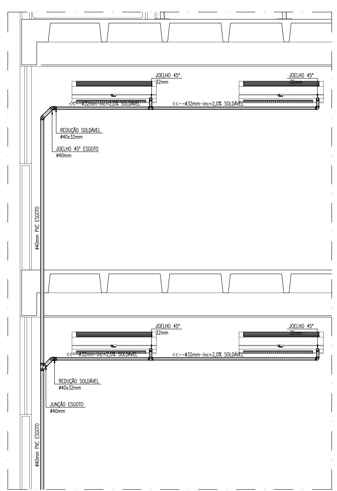
DETALHE INTERLIGAÇÃO DRENOS ESCALA: 1/25
