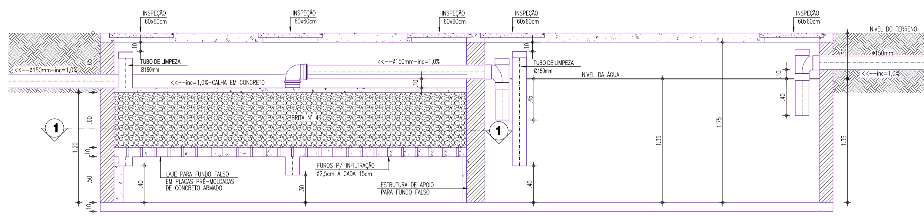
CORTE AA - TANQUE SÉPTICO / FILTRO ANAERÓBICO ESCALA : 1/25
