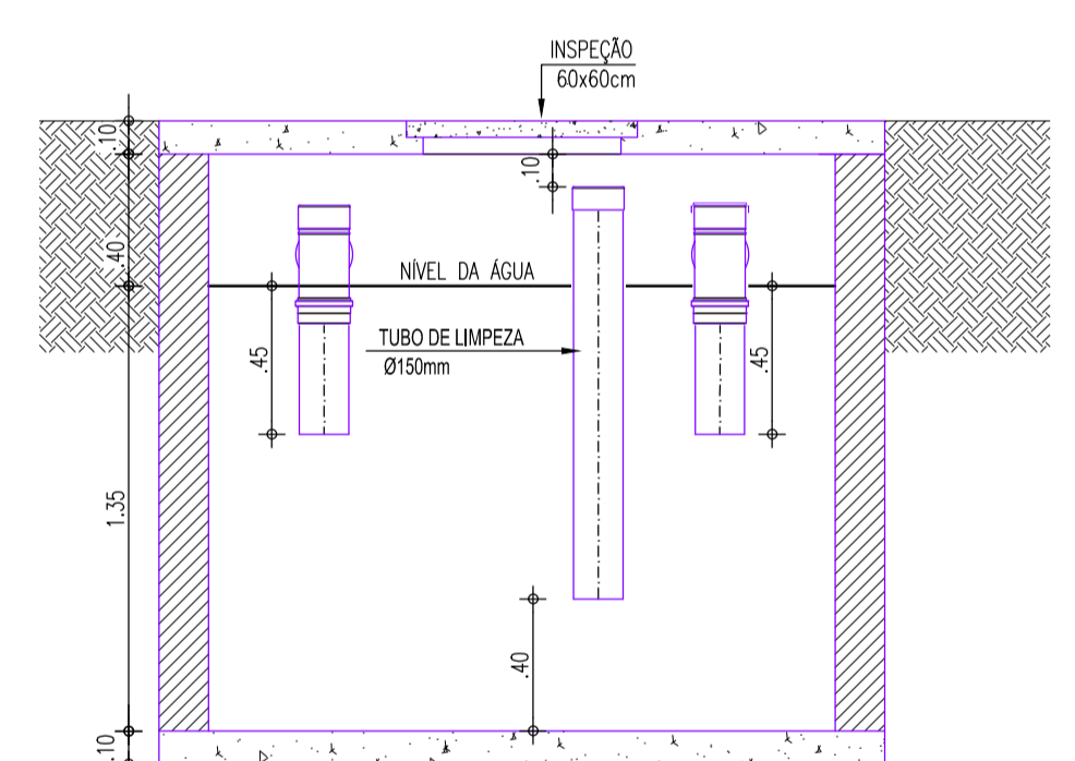
CORTE BB - TANQUE SÉPTICO ESCALA : 1/25
