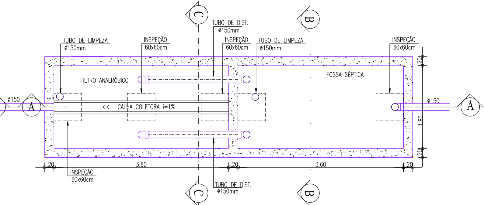
PLANTA BAIXA FOSSA SÉPTICA/FILTRO ANAERÓBICO/SUMIDOURO ESCALA : 1/50
