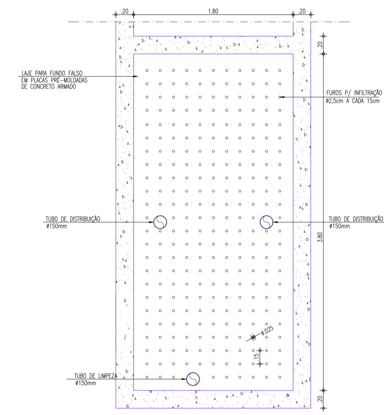
FUNDO FALSO - FILTRO ANAERÓBICO ESCALA : 1/25
