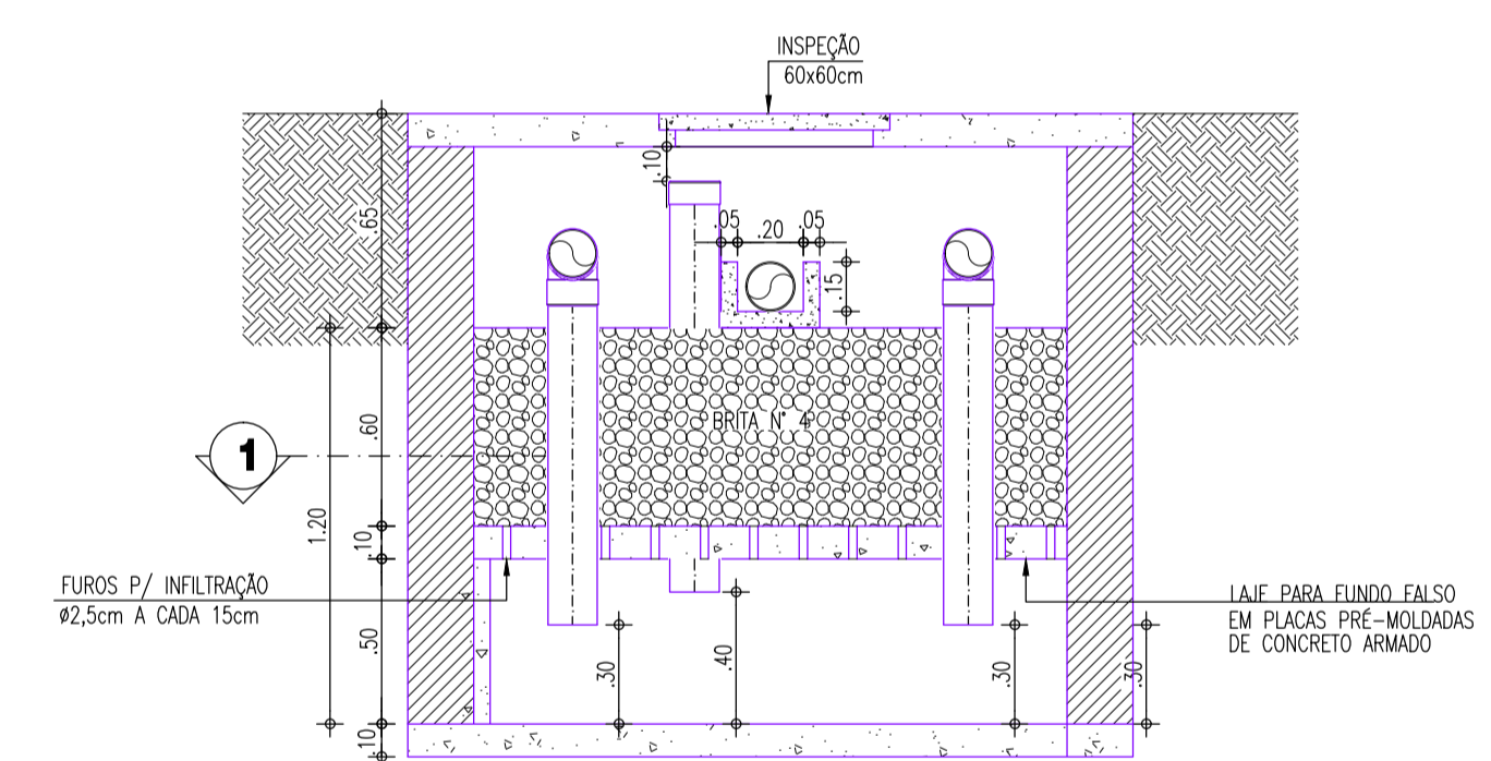
CORTE CC - FILTRO ANAERÓBICO ESCALA : 1/25
