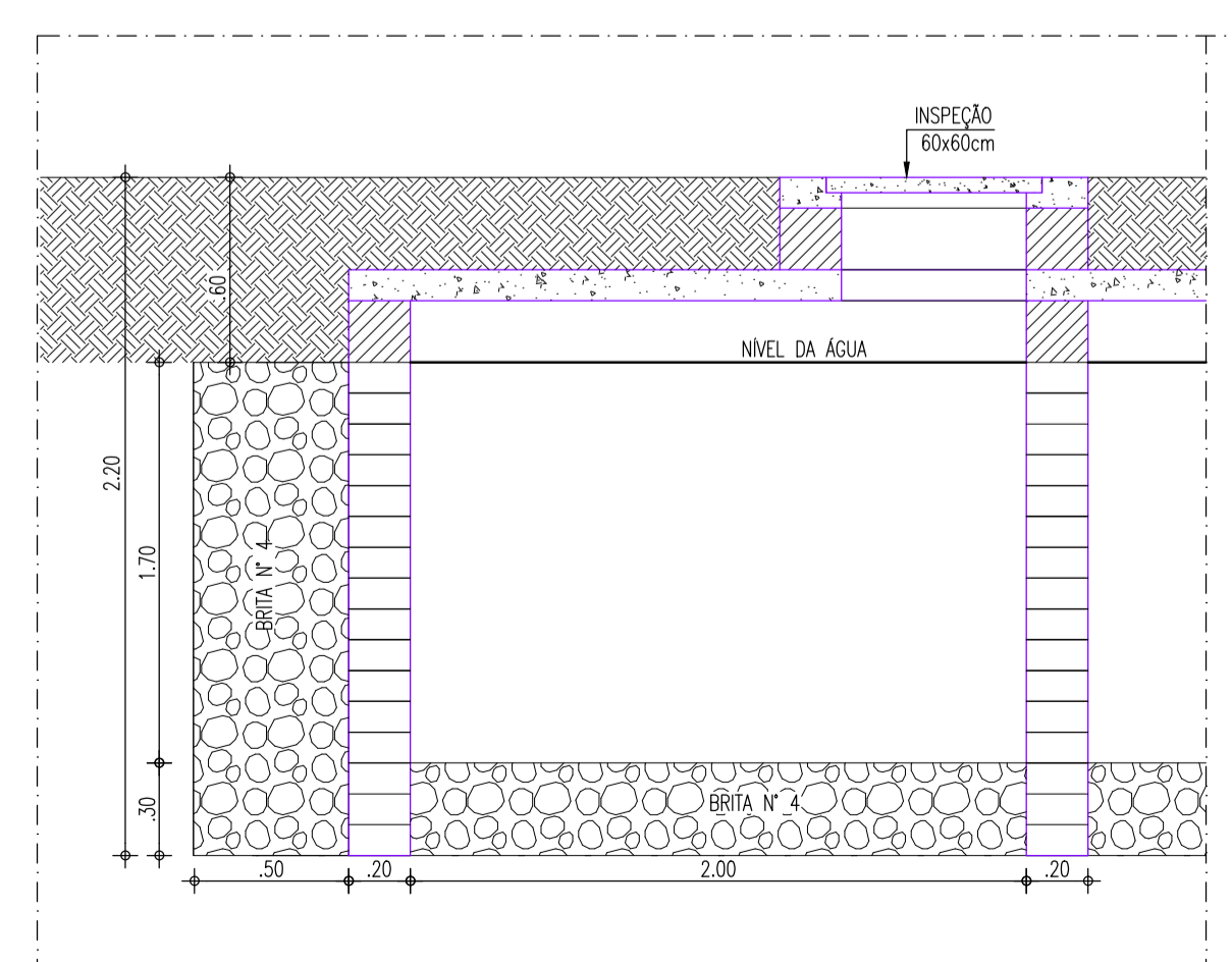
CORTE BB - SUMIDOURO ESCALA : 1/25
