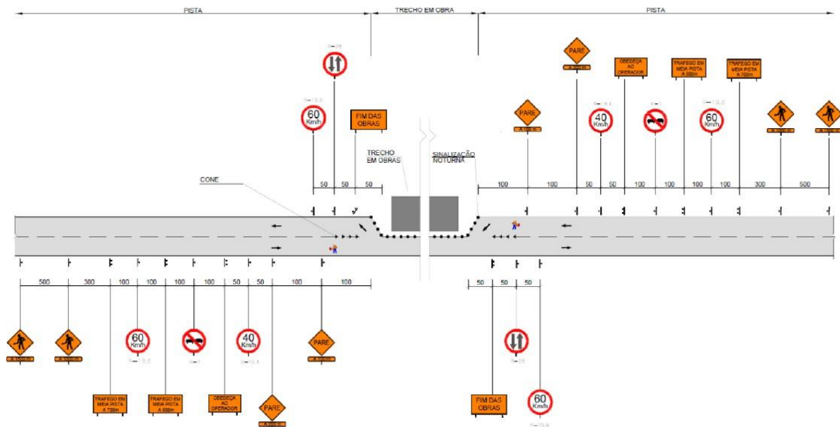
Figura 10 – Modelo de esquema de sinalização para interrupção parcial de tráfego
