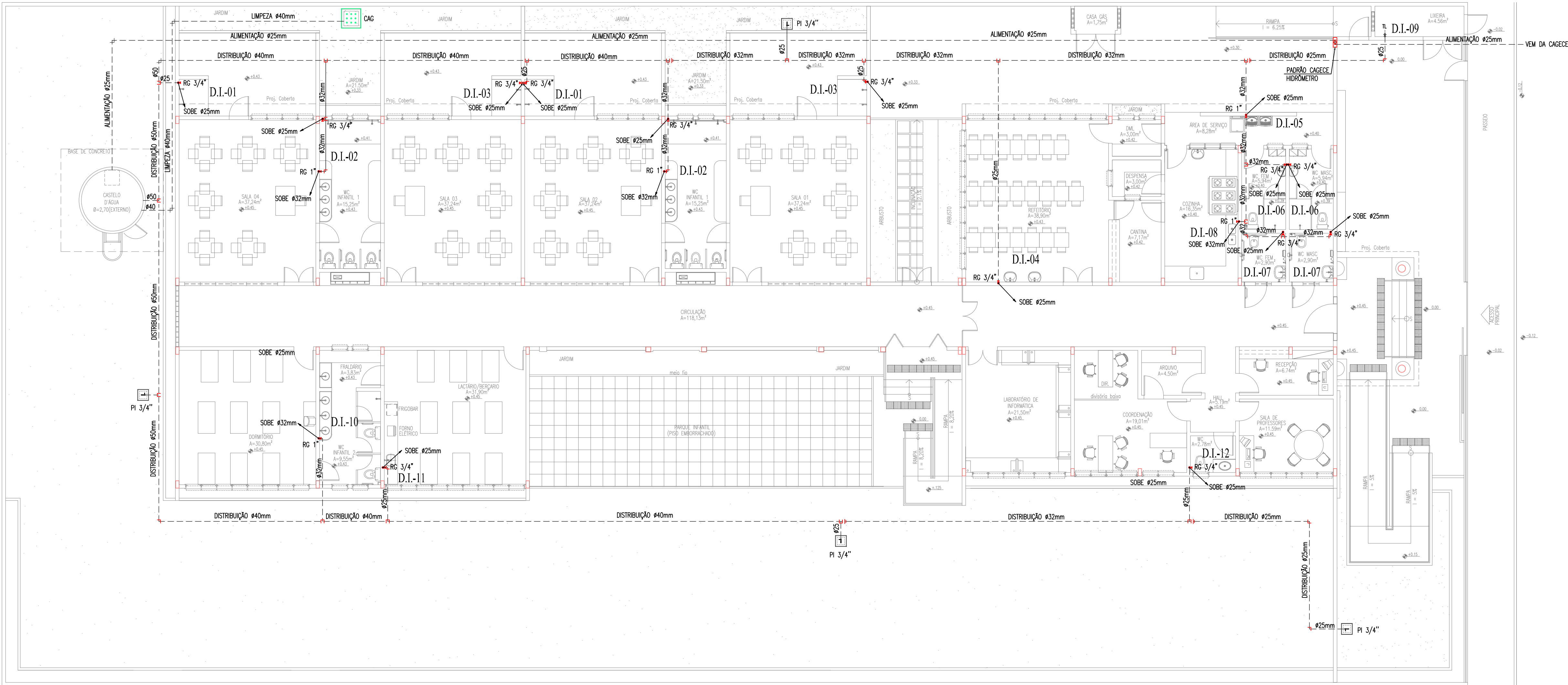
PLANTA BAIXA - PAV. TÉRREO ESCALA : 1/100
