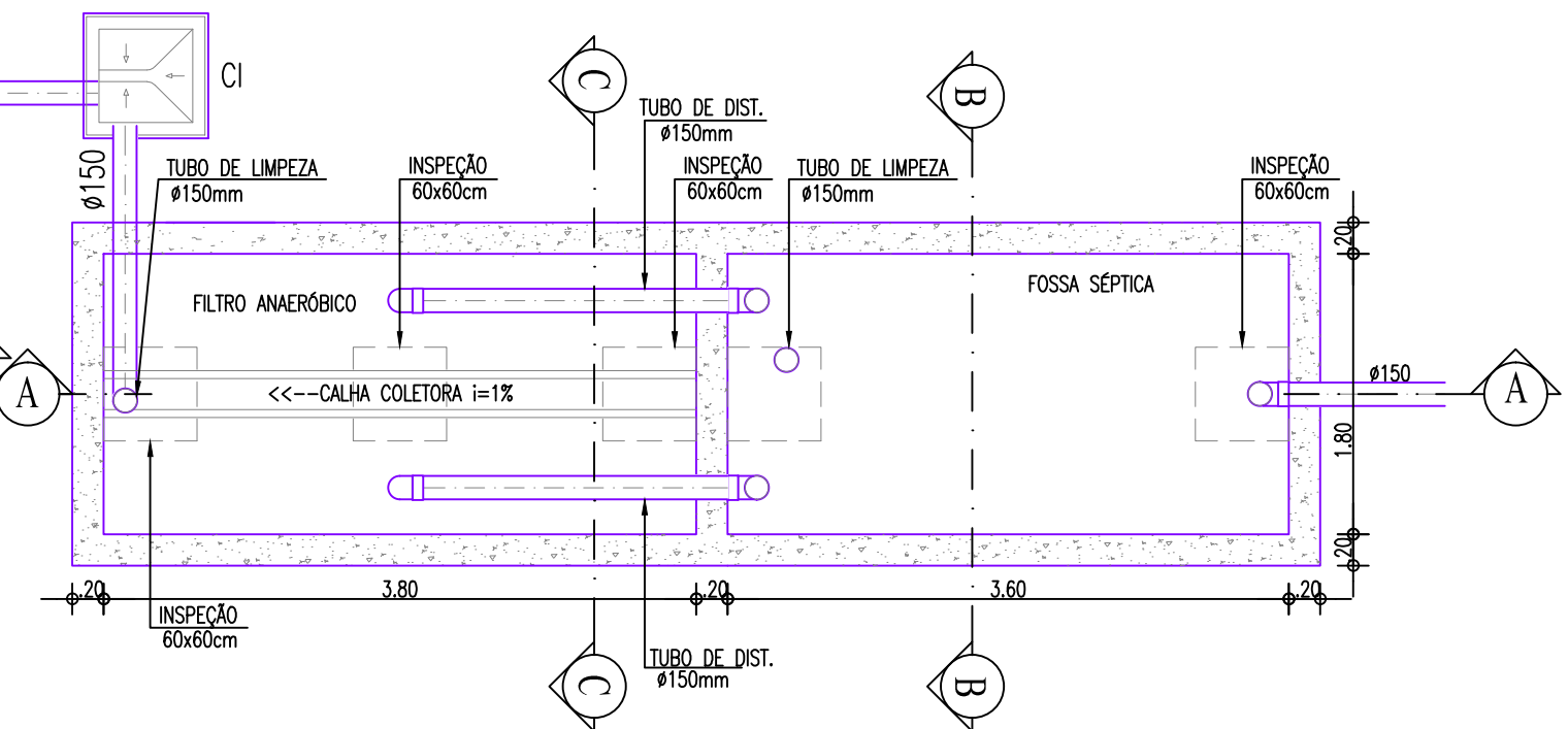
PLANTA BAIXA - FOSSA SÉPTICA/FILTRO ANAERÓBICO/SUMIDOURO ESCALA : 1/50
