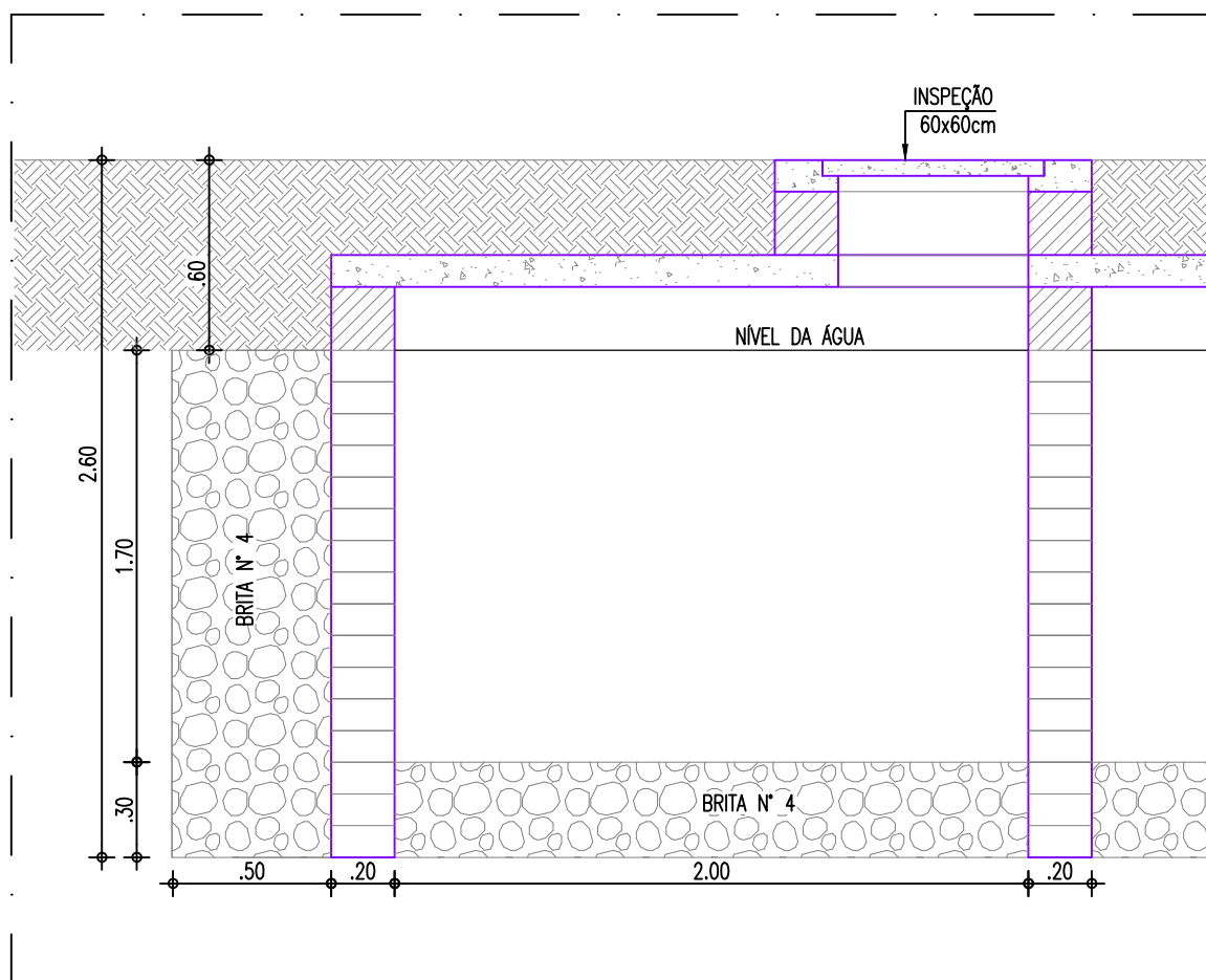
CORTE BB - SUMIDOURO ESCALA : 1/25
