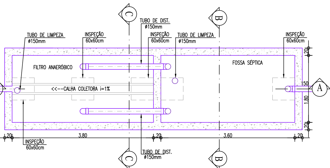
PLANTA BAIXA - FOSSA SÉPTICA/FILTRO ANAERÓBICO
